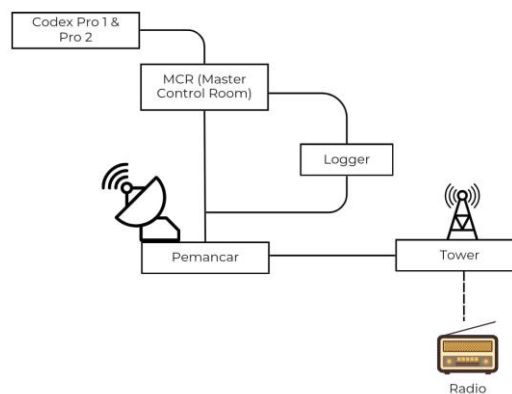
Gambar 1. Sistem Penyiaran Programa 1(94.6 FM) dan Programa 2 (101.6 FM)
