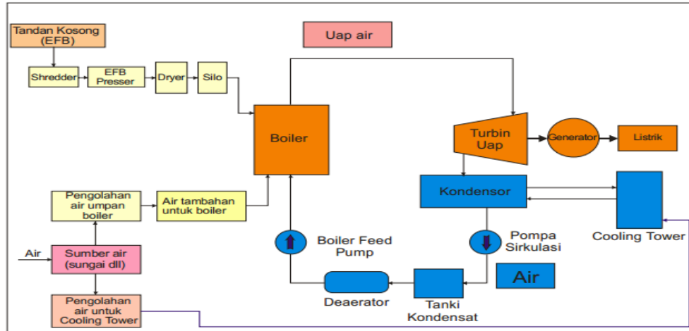
Gambar 4 Skema Pembangkit Listrik Tenaga Biomassa Sawit (PLTBS) (Febijanto 2011)
