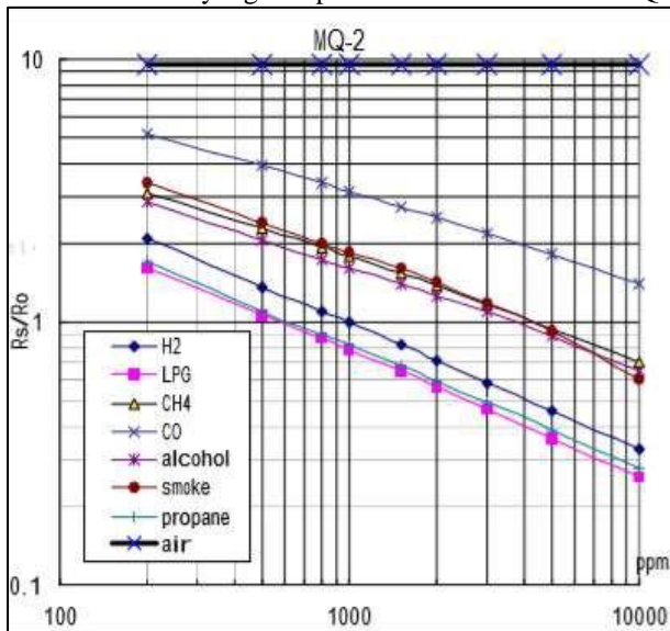
Gambar 4 karakteristik sensivitas MQ2 Sumber : Datasheet MQ2
