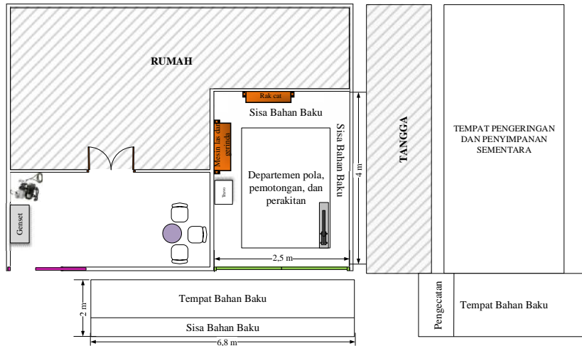
Gambar 1. Layout awal Bengkel Pras Las
